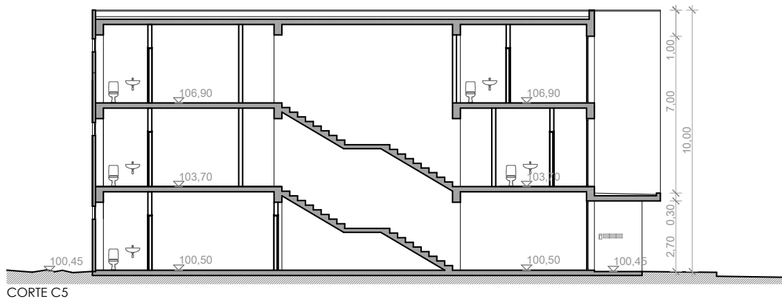
CORTE C5
