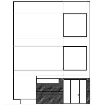
ALÇADO NASCENTE
