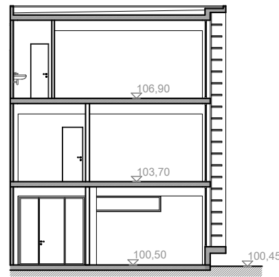
CORTE C2
