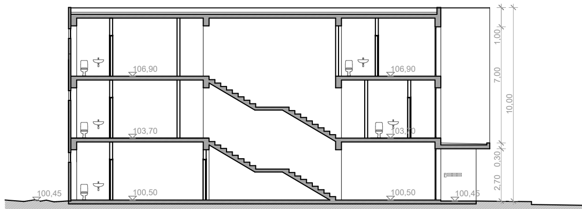
CORTE C5
