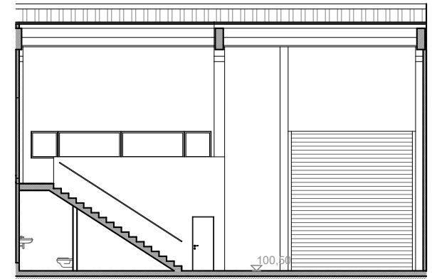
CORTE C2
