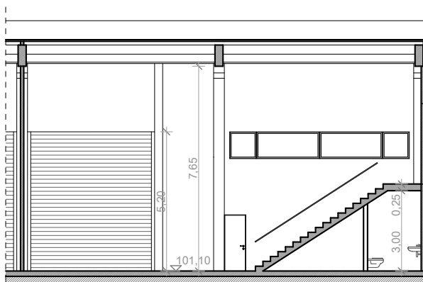
CORTE C1
